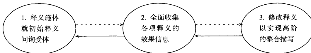
释义施体的“自适应”示意图
